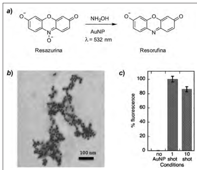
FIGURA 7. a) Reducció de la resazurina a resorufina en presència d'hidroxilamina i AuNP, a temperatura ambient i amb irradiació amb llum verda polsada ( \lambda = 532 nm). b) Imatge de TEM de les AuNP emprades (diàmetre \sim 13 nm). c) Conversió de la reacció de reducció en absència de fotocatalitzador (no AuNP) i en presència de AuNP i amb irradiació amb 1 pols (1 shot) i 10 polsos (10 shot) de llum verda. La conversió del procés s'expressa com l'increment relatiu del senyal de fluorescència mesurat respecte del 100 % de resorufina. Adaptat de [19] amb el permís de la Royal Society of Chemistry.
