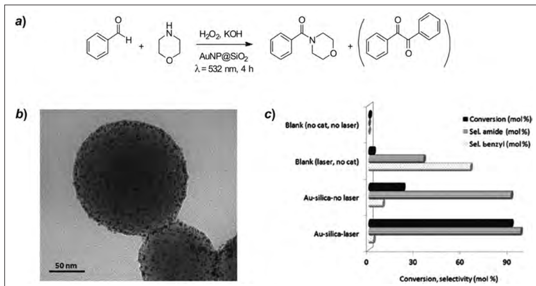
FIGURA 8. a) Reacció d'amidació entre el benzaldehid i la morfolina fotocatalitzada per AuNP@SiO 2 a temperatura ambient i sota irradiació amb llum verda contínua ( \lambda = 532 nm). A les condicions emprades, el dibenzoil es pot generar com a subproducte. b) Imatge de TEM del fotocatalitzador emprat, que consisteix en AuNP de ~2 nm de diàmetre suportades sobre nanopartícules de SiO 2 de ~150 nm de diàmetre. c) Conversió i selectivitat de la reacció d'amidació en absència i en presència de fotocatalitzador i irradiació. Adaptat de [28] amb el permís de la Royal Society of Chemistry.
