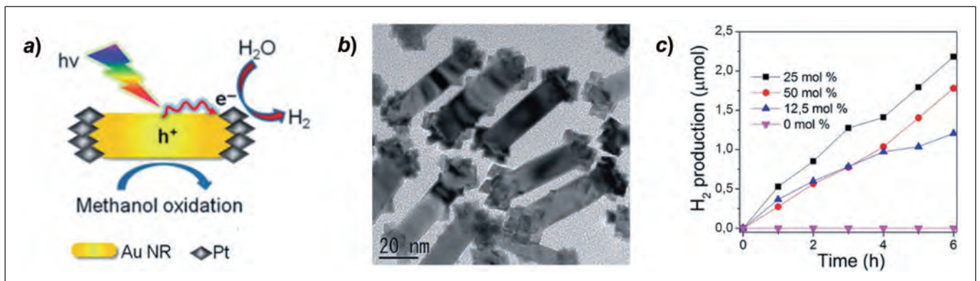
FIGURA 6. a) Generació de \text{H}_2 en barreges aqua: metanol a temperatura ambient utilitzant irradiació contínua amb llum visible ( \lambda = 460\text{--}820 \text{ nm} ) i «nanorods» d'or (longitud \sim 50 \text{ nm} , diàmetre \sim 13 \text{ nm} ) funcionalitzats als extrems amb nanopartícules piramidals de Pt (aresta \sim 7 \text{ nm} ) com a fotocatalitzadors. b) Imatge de microscòpia electrònica de transmissió (TEM) dels fotocatalitzadors emprats. c) Producció de \text{H}_2 sota irradiació contínua per a fotocatalitzadors amb diferent contingut de Pt (0–25 mol %). Adaptat de [20] amb permís. Copyright 2014 American Chemical Society.
