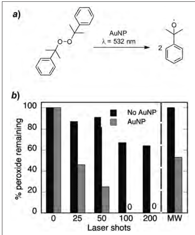
FIGURA 5. a) Reacció de dissociació del peròxid de dicumil després d'irradiar amb llum làser polsada a \lambda = 532 \text{ nm} en presència de AuNP. b) Percentatge de substrat no reaccionat respecte al nombre de polsos de llum làser aplicats a solucions 1 mM de peròxid de dicumil en \text{H}_2\text{O} amb un 5 % de metanol. Adaptat de [32] amb permís. Copyright 2011 American Chemical Society.
